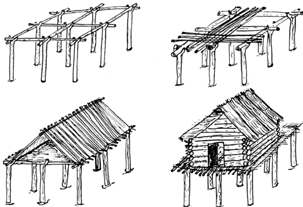
Рис.23. Реконструкция хозяйственного амбара.
