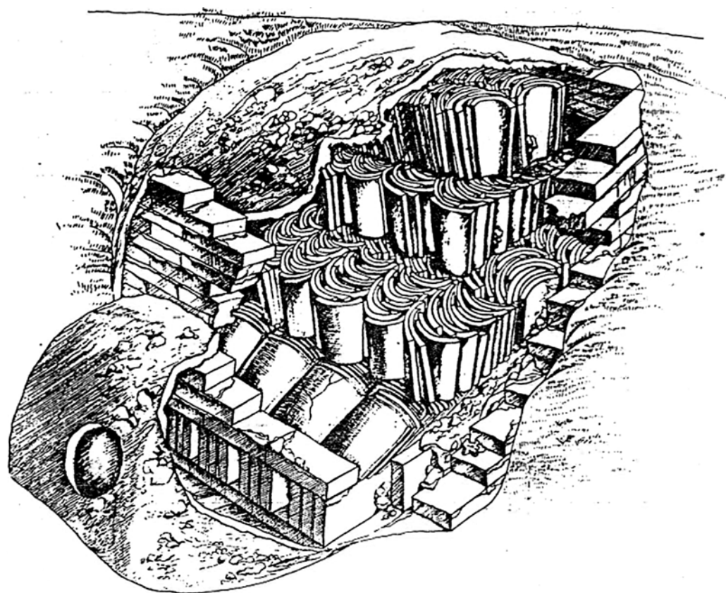
Рис.8. Черепичная печь.
