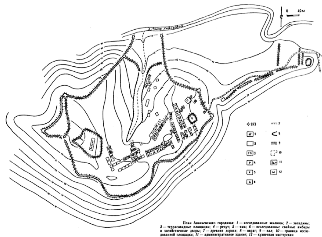
Рис. 17. План Ананьевского городища (по В.А. Хореву).
